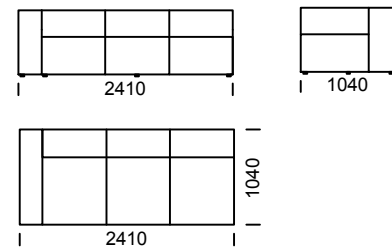
Siedzisko B3 / Seat B3 / Sitzfläche B3
