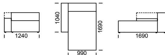
Szezlong 2 / Chaise longue 2 / Chaiselongue 2
