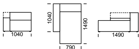
Szezlong 1 / Chaise longue 1 / Chaiselongue 1
