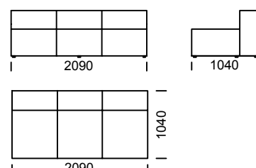
Siedzisko centralne C3 / Central seat C3 / Mittelsitz C3
