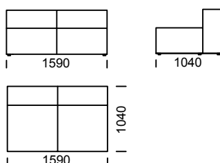
Siedzisko centralne C2 / Central seat C2 / Mittelsitz C2
