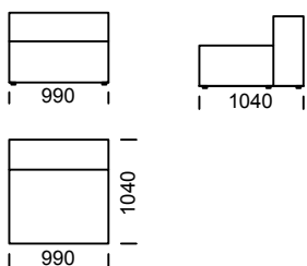
Siedzisko centralne C1 / Central seat C1 / Mittelsitz C1
