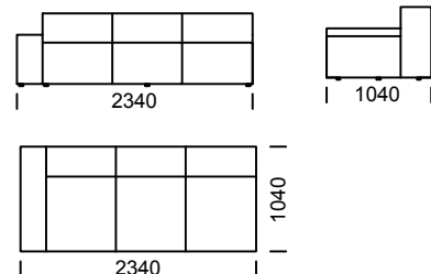
Siedzisko A3 / Seat A3 / Sitzfläche A3
