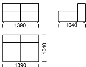
Siedzisko centralne C1 / Central seat C1 / Mittelsitz C1
