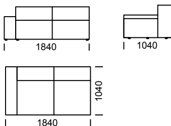
Siedzisko A2 / Seat A2 / Sitzfläche A2
