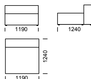
Siedzisko centralne C3 / Central seat C3 / Mittelsitz C3
